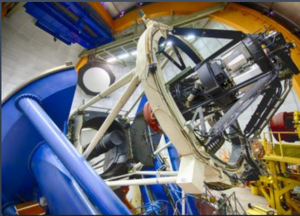
Dark Energy Survey
